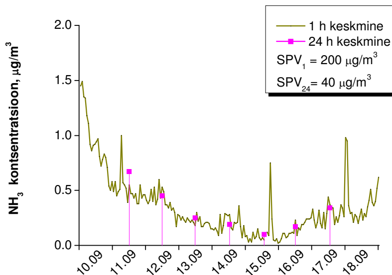
Joonis 8 NH 3 keskmine kontsentratsioon
