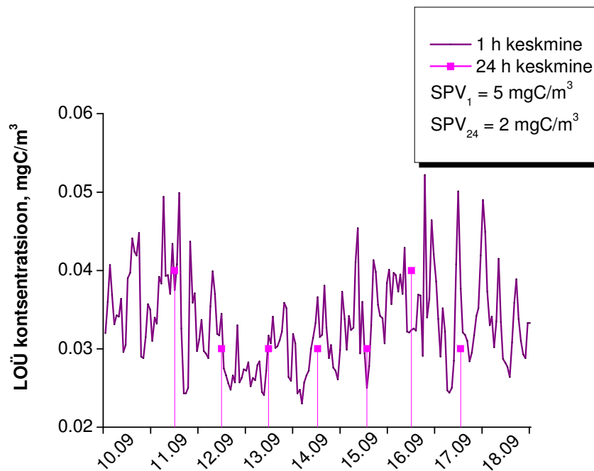
Joonis 6 LOÜ keskmine kontsentratsioon
