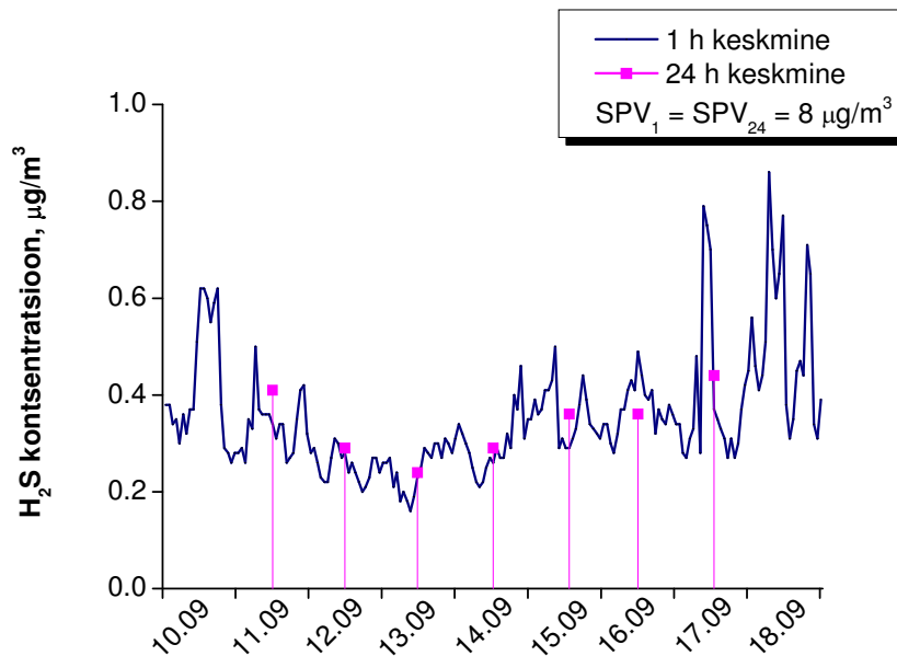
Joonis 7 H 2 S keskmine kontsentratsioon
