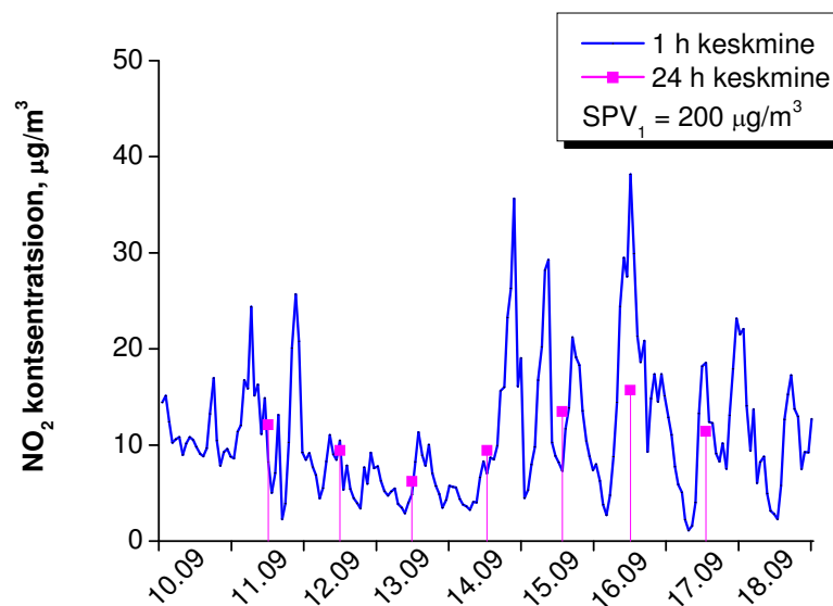
Joonis 5 NO 2 keskmine kontsentratsioon
