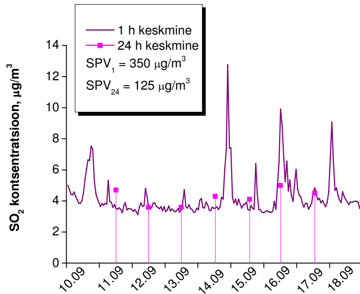
Joonis 9 SO 2 keskmine kontsentratsioon
