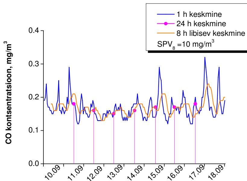
Joonis 3 CO keskmine kontsentratsioon
